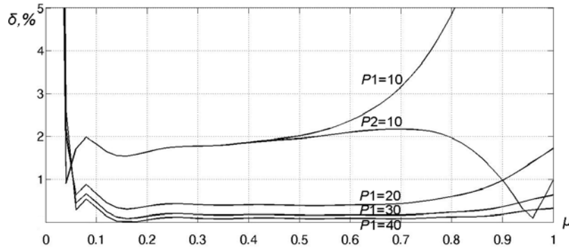
Рис. 1. Графіки залежностей відносної похибки \delta значень суми квадратів вищих гармонік відносно значень глибини модуляції \mu для різних значень параметру кратності модуляції P
