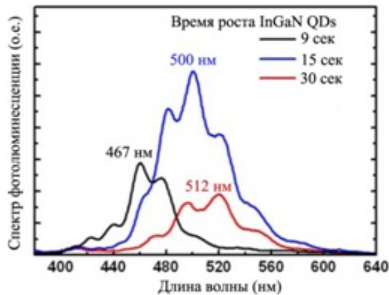
Рис. 2. Графики спектра фотолюминесценции InGaN квантовых точек, измеренный при комнатной температуре с временами роста 9, 15 и 30 с
