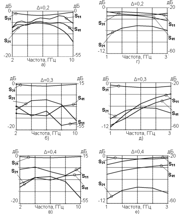
Рис. 4. Частотные зависимости элементов [S] структуры с полукруглыми внутренними проводниками при различных расстояниях Δ между ними (а, б, в – изгиб согласно рис. 2 а; г, д, е – изгиб согласно рис. 2 б)
