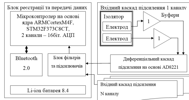
Рис. 1. Загальна структура розробленої системи реєстрації сигналу поверхневої ЕМГ
