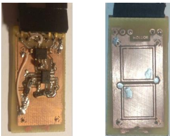
Рис. 3. Зовнішній вигляд вхідного каскаду та диференціальної пари електродів
