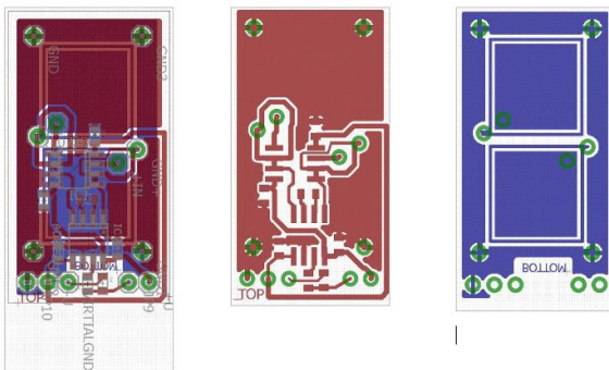
Рис. 2. Топологія друкованої плати вхідного каскаду
