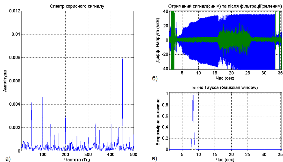
Рис. 6. Спектр корисного сигналу на 8 секундi при розслабленому м'язi, отриманий i відфільтрований сигнал та положення вікна в момент розрахунку спектру. а) Спектр сигналу при розслабленому м'язi, б) отриманий сигнал - синім кольором, після фільтрації - зеленим, в) положення вікна Гаусса для розрахунку спектру сигналу
