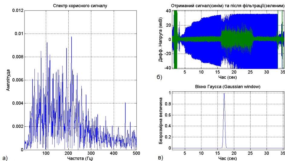
Рис. 7. Спектр корисного сигналу на 17 секунд при напруженому м'язі, отриманий і відфільтрований сигнал та положення вікна в момент розрахунку спектру. а) Спектр сигналу при розслабленому м'язі, б) отриманий сигнал - синім кольором, після фільтрації - зеленим, в) положення вікна Гаусса для розрахунку спектру сигналу
